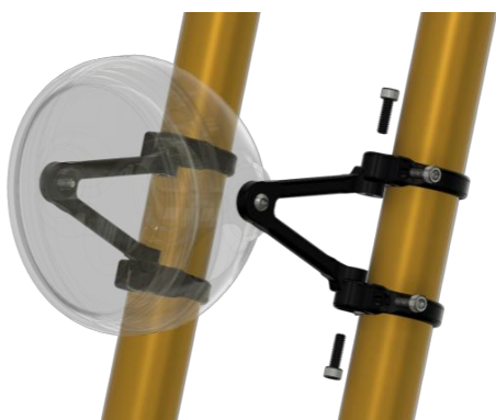
Montage Beispiel für den Lampenhalter 1, 2, 3
